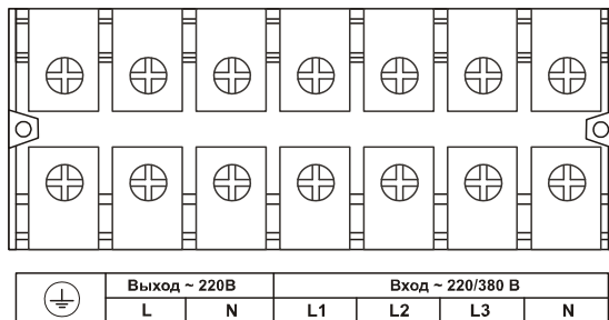
Рисунок 11 – Внешний вид клеммных блоков ИБП ATS 30000 3/1 T-X, ИБП ATS 30000 3/1 T-BX
