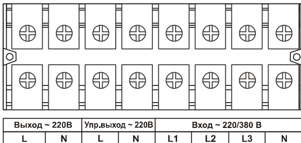
Рисунок 8 – Внешний вид клеммных блоков ИБП ATS 10000 3/1 T-VX, ИБП ATS 10000 3/1 T-X
