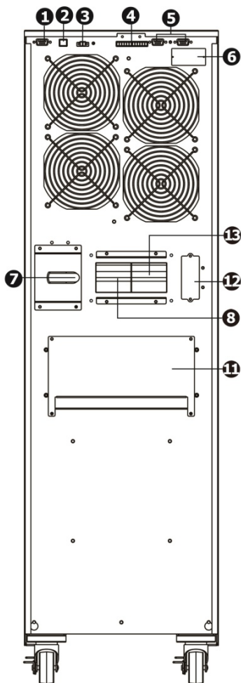
Рисунок 7 - Задняя панель ИБП ATS 30000 3/1 T-VX
