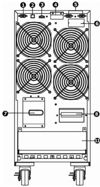
Рисунок 4 - Задняя панель ИБП ATS 15000 3/1 T-X, ATS 20000 3/1 T-X
