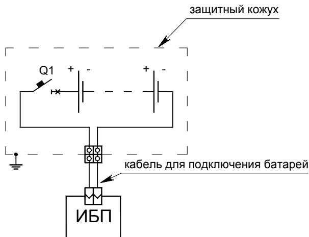
Рисунок 12 – Схема электрическая подключения аккумуляторных батарей к ИБП
