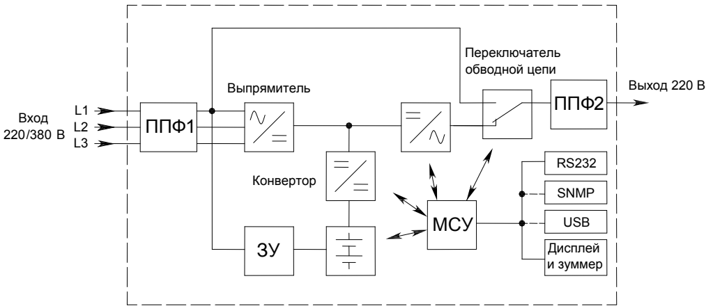
Рисунок 1 - Структурная схема ИБП
