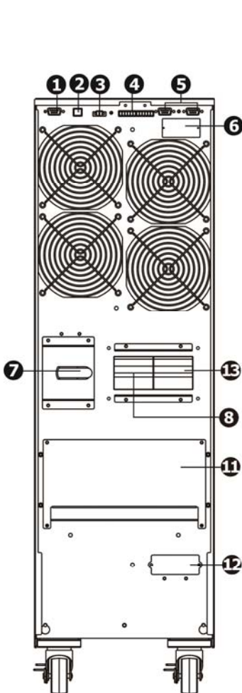
Рисунок 6 - Задняя панель ИБП ATS 30000 3/1 T-X
