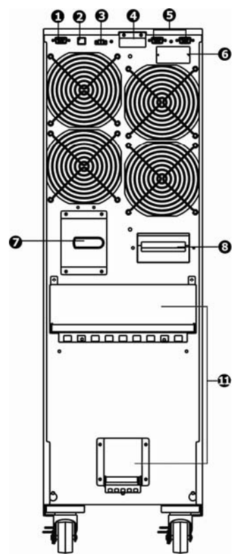
Рисунок 5 - Задняя панель ИБП ATS 15000 3/1 T-BX, ATS 20000 3/1 T-BX
