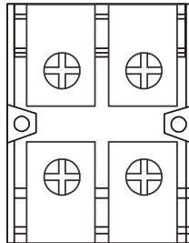
Рисунок 10 – Внешний вид клеммных блоков ИБП ATS 15000 3/1 T-BX, ИБП ATS 20000 3/1 T-BX
