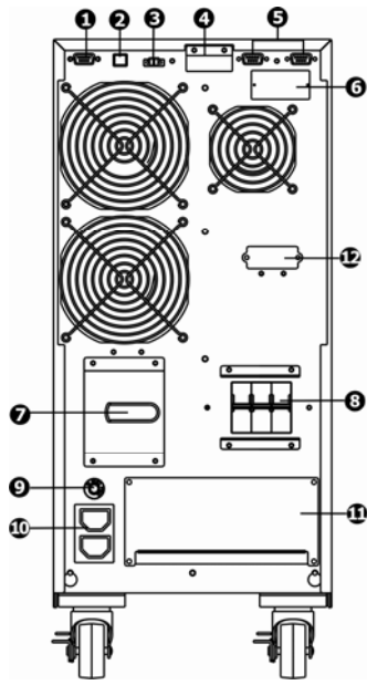
Рисунок 3 - Задняя панель ИБП ATS 10000 3/1 T-BX, ATS 10000 3/1 T-X
