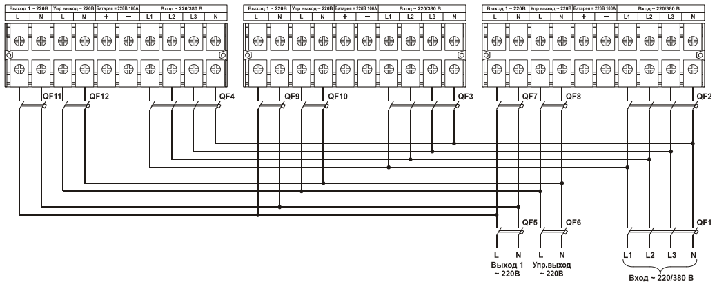
Рисунок 31 – Соединение входов и выходов трех ИБП в параллельной системе
