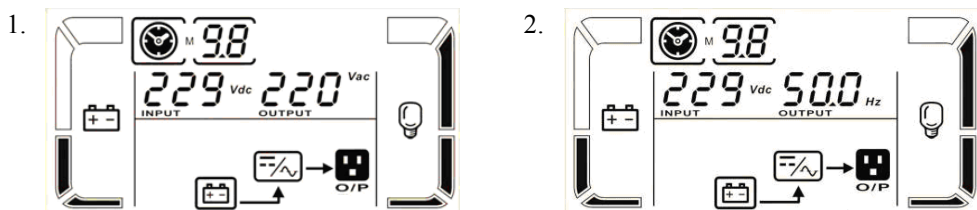
Рисунок 21 – Показания LCD-дисплея ИБП в автономном режиме
