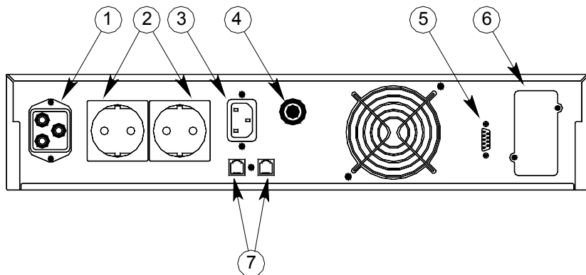
Рисунок 3 - Задняя панель ИБП ATS 1000 R, ATS 1000 R-B
