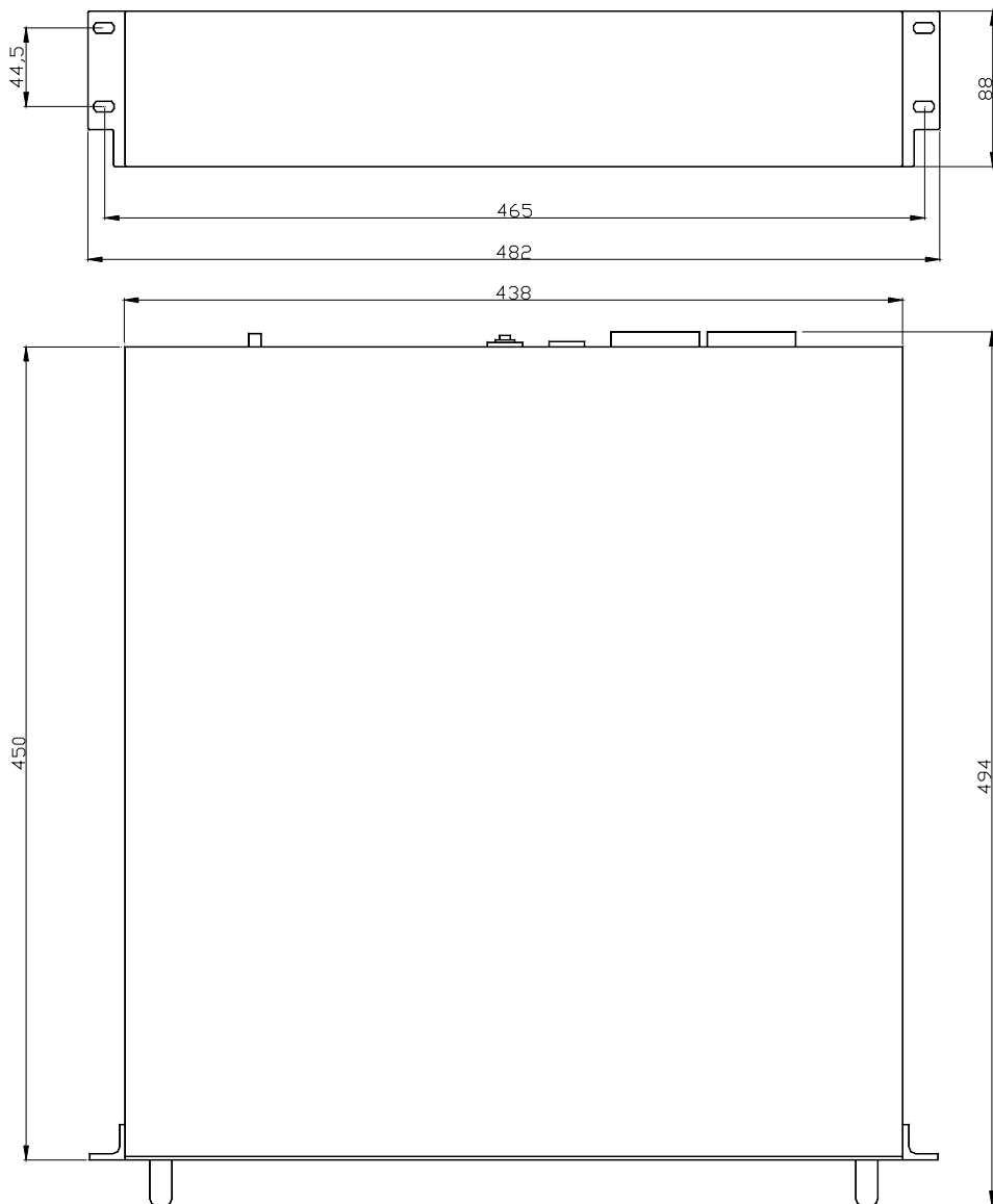
Рисунок А.1 – Габаритные и установочные размеры ИБП
