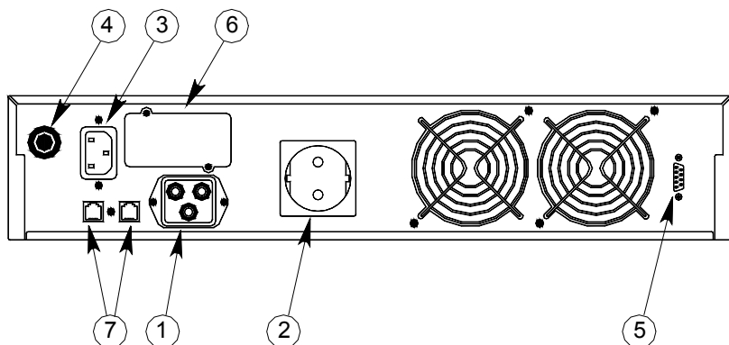
Рисунок 4 - Задняя панель ИБП ATS 2000 R, ATS 2000 R-B, ATS 3000 R-B
