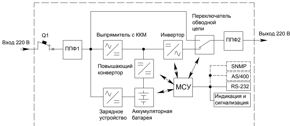
Рисунок 1 - Структурная схема ИБП
