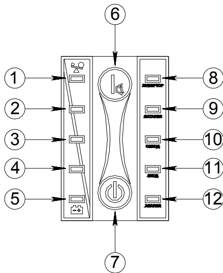
Рисунок 2 - Расположение органов управления и индикации на передней панели ИБП
